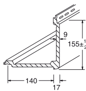
Universal angle 1)
